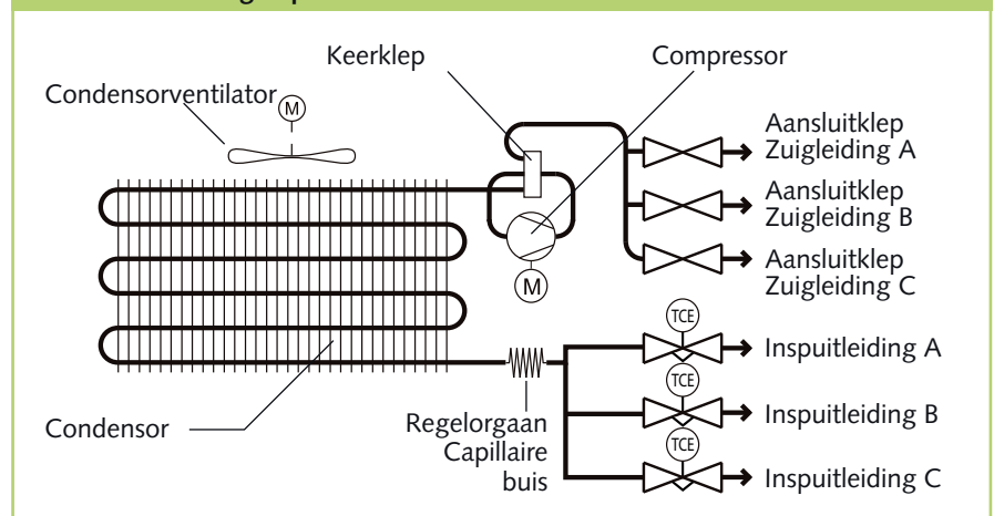
Schema koudekringloop buitenunit MVT 900DC
