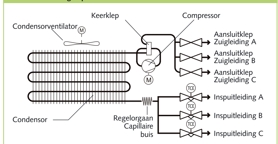
Schema koudekringloop buitenunit
