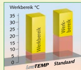
Inzet voor ontvochtigen bij LowTEMP uitvoering al vanaf 6 °C mogelijk
