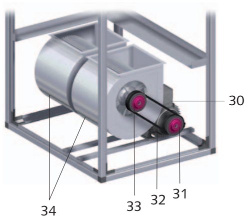
Abb. Ventilator mit Riemenantrieb
